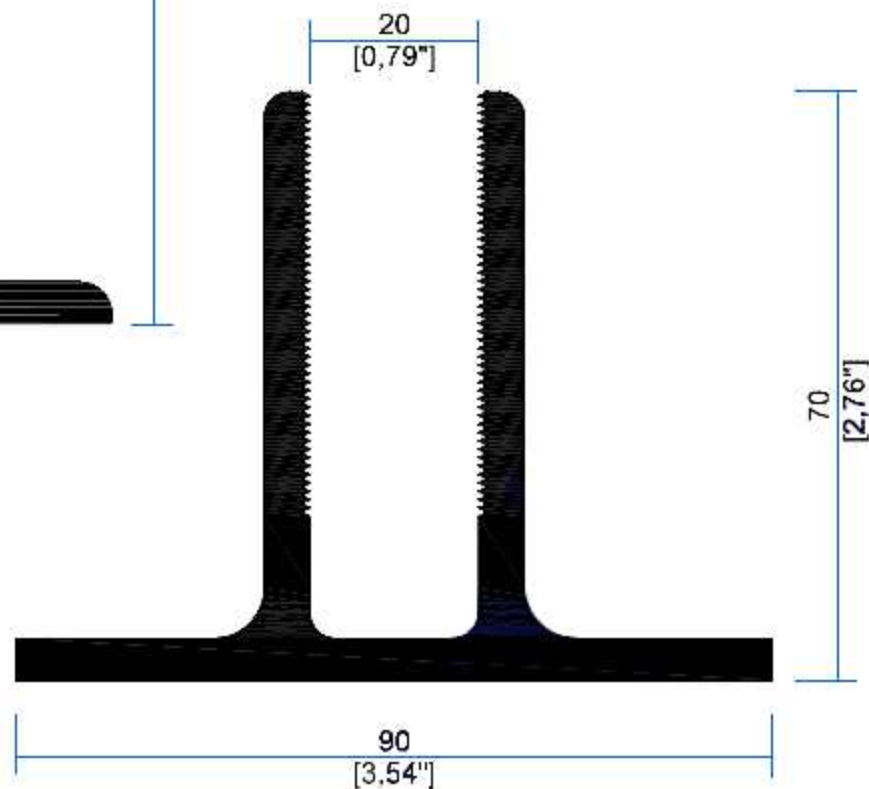
V21105 Zoclo para Pasamano 2 3/4"
