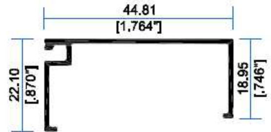
6606 Junquillo
