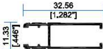
3358 Zapata
