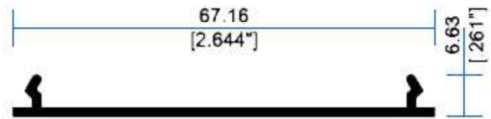
32563 Tapa Lisa
