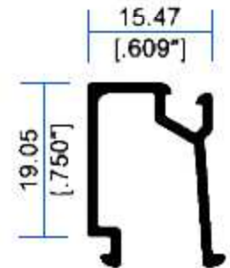
12543 Junquillo Recto
