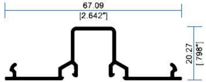
42505 Tapa Bolsa
