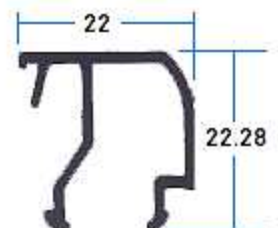
6029 Junquillo Curvo
