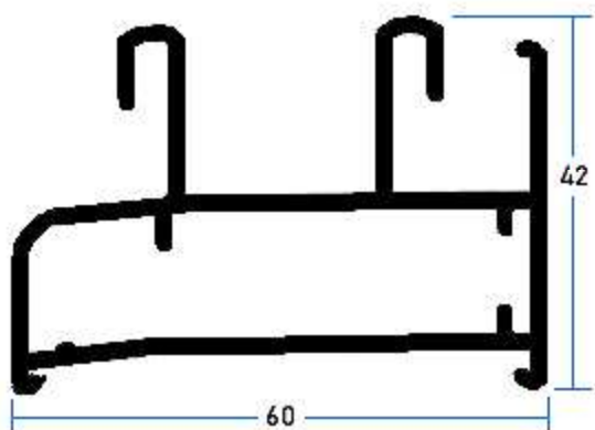
107003 Riel Perimetral 2 Vias
