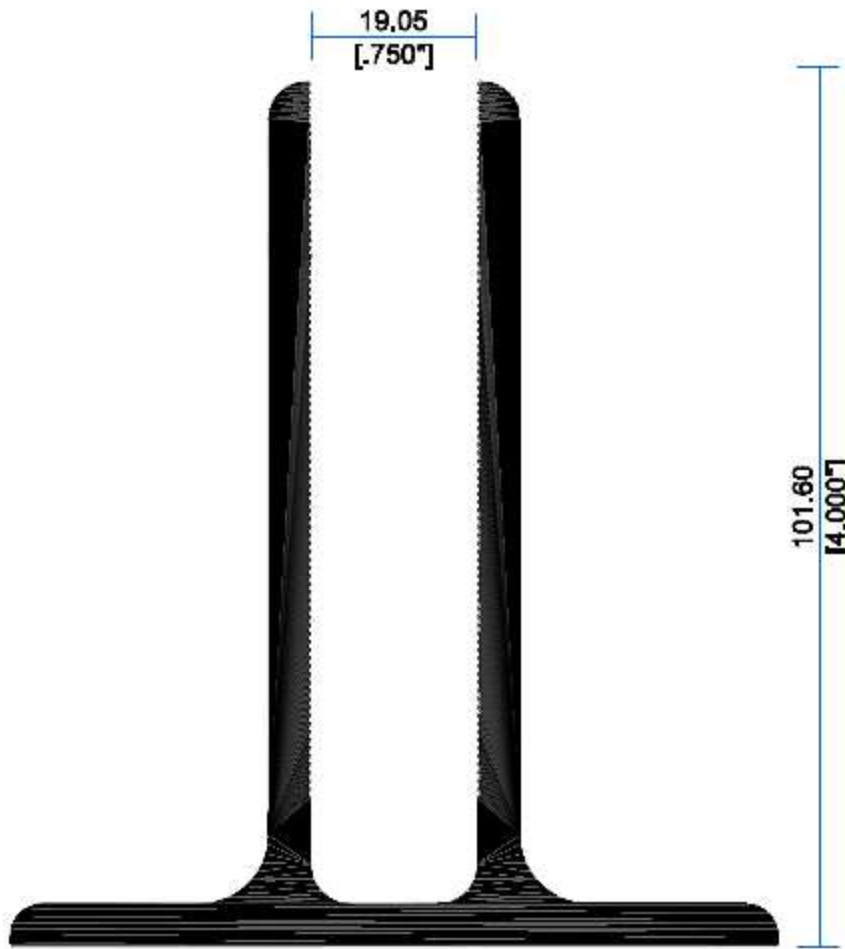
20293 Zoclo para Pasamano 4"
