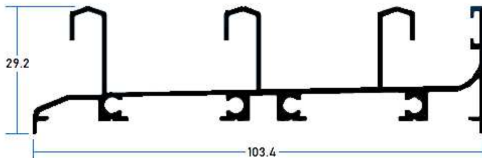
B10587 Riel 3 Vias
