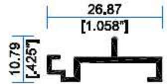
9966 Adaptador
