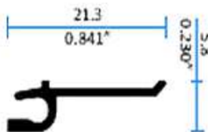
2324 Guarda Polvo
