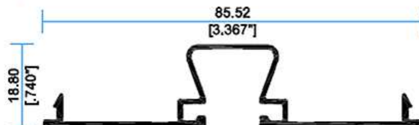
6609 Tapa Bolsa
