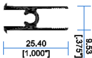
7949 Horizontal
