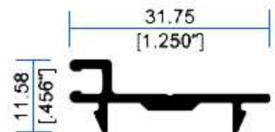
13638 Adaptador Mosquitero
