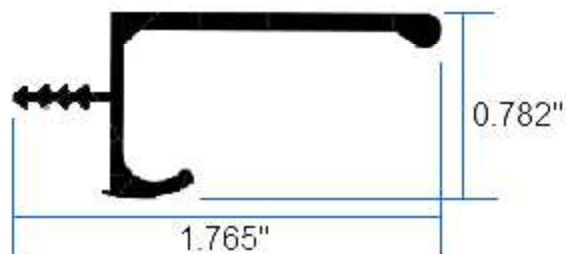
32102 Jaladera Tipo J
