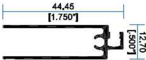
6533 Horizontal
