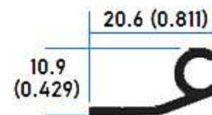
35002 Sellapolvo Auto Hembra
