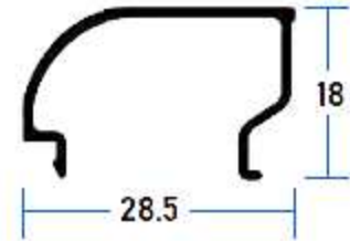
1433 Junquillo Redondo
