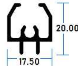
2415 Recercado
