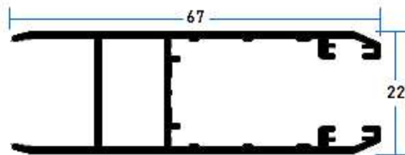
107002 Hoja Perimetral Doble Vidrio
