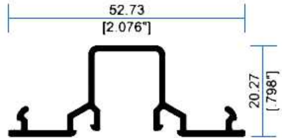
12505 Tapa Bolsa
