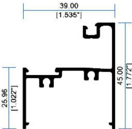
12608 Escalonado
