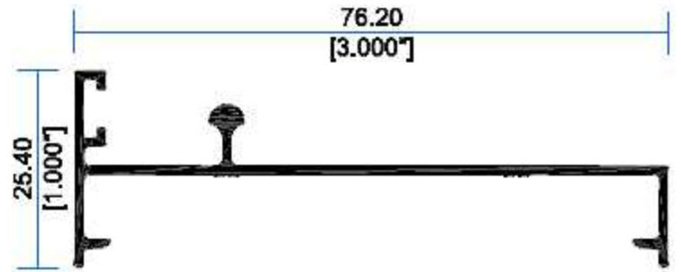
9957 Riel
