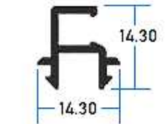
4610 Adaptador Mosquitero
