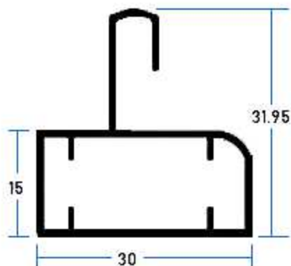
79666 Riel Adaptador
