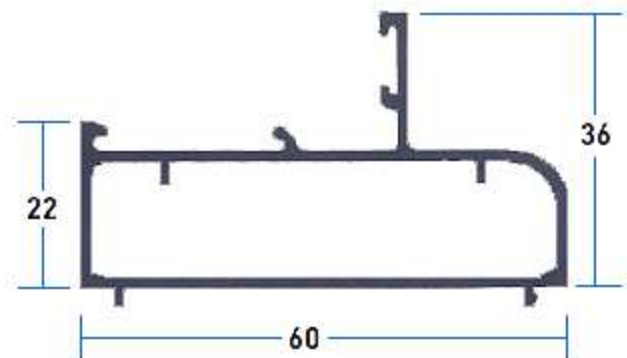
3510 Fijo Tubular
