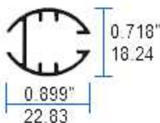
31453 Contrapeso Ovalado
