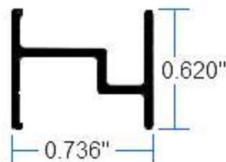
E2204 Intermedio
