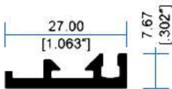
5173 Pesada
