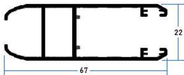
107001 Hoja Perimetral
