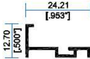
7013 Portavidrio
