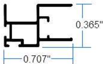
E2203 Cerco Jaladera
