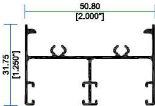
7518 Jamba
