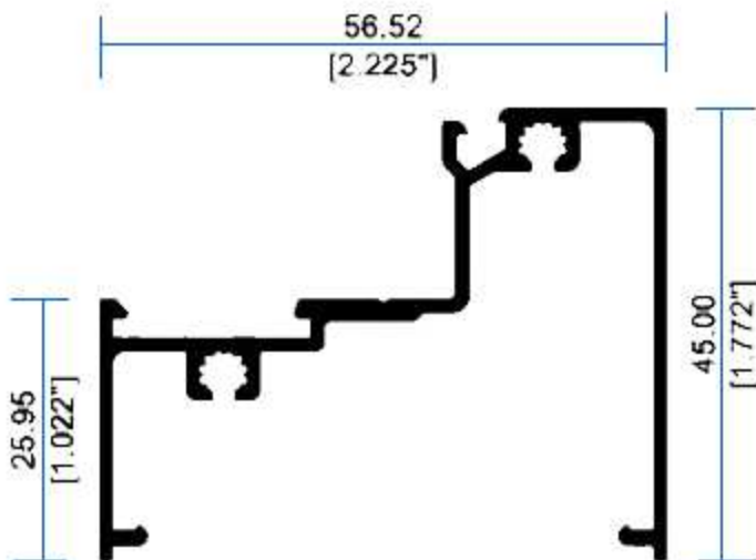
12506 Escalonada
