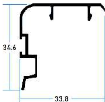
10513 Traslape Corto
