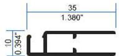
3536 Hoja Rueda Mosquitero
