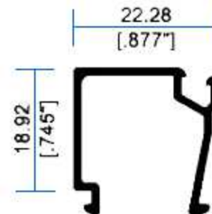
12507 Junquillo
