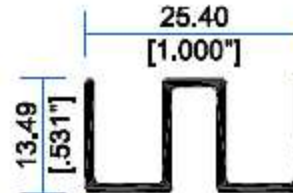
3329 Guia Doble
