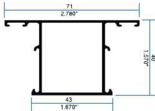
11405 Pilastra Puerta
