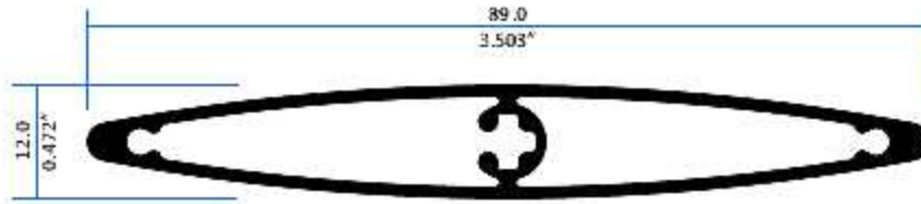
6053 Rompe Vista 3 1/2"
