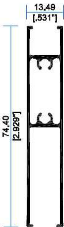
7825 Zoclo Puerta
