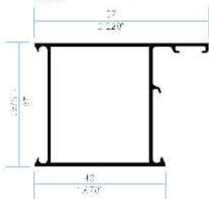
11407 Cercos Lisa Puerta
