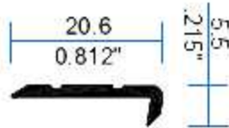
3150 Ribete Decorativo 3/4"
