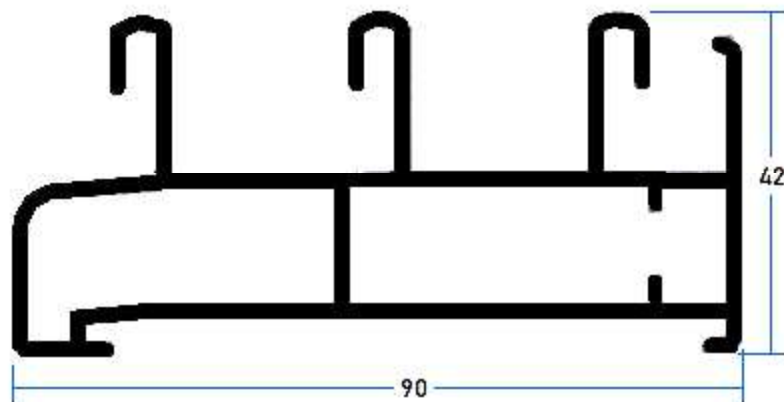
107004 Riel Perimetral 3 Vias
