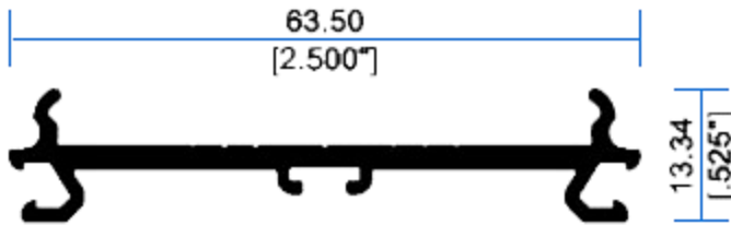
14350 Moldura Union
