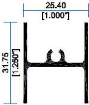
9958 Cabezal Duo
