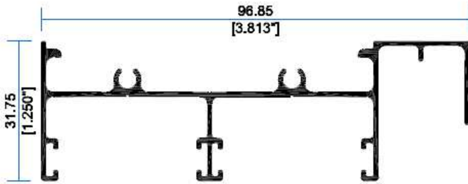
9272 Riel C/Mosquitero exterior
