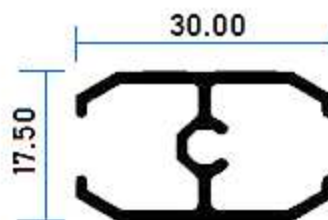
2416 Cuadricula Española
