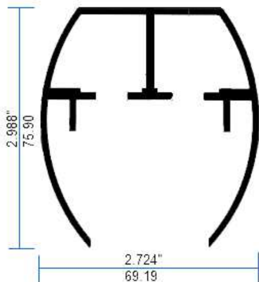
10478 Riel Superior 6mm Redondo
