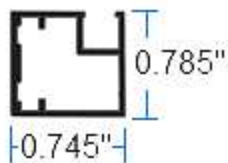
10667 Puerta Junior
