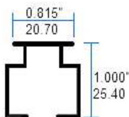
31456 Riel Cortinero Hotelero
