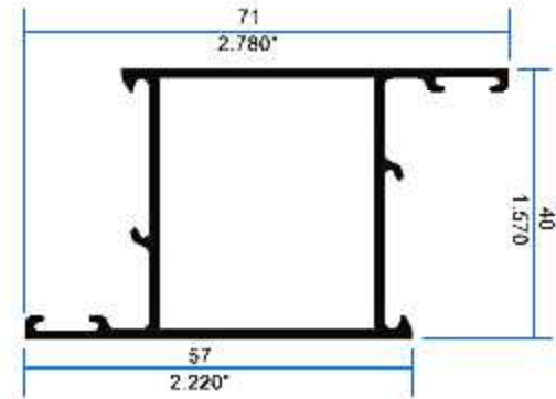
11406 Hoja Lisa Puerta
