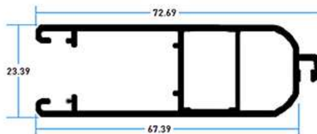
Hoja Mosquitero
