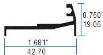
107205 Riel Inferior 9mm
