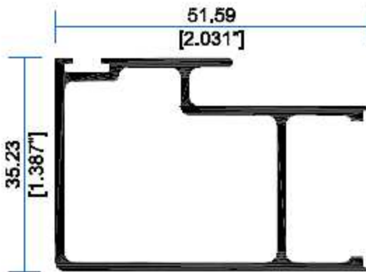
9963 Traslape Ventana Duo
