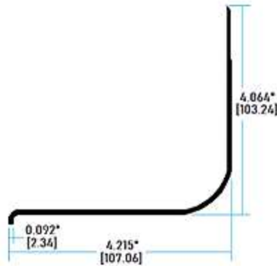
32198 ESQUINERO CARROCERO CHICO
