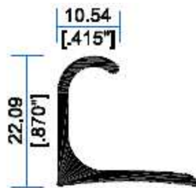
4154 Jaladera Trompa de Elefante
