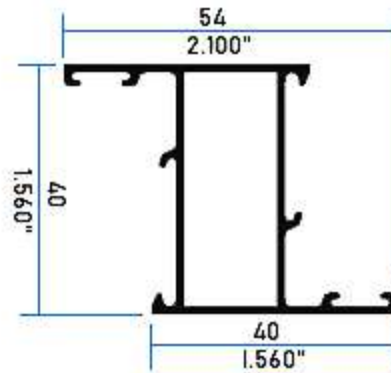
11401 Hoja Lisa Ventana
