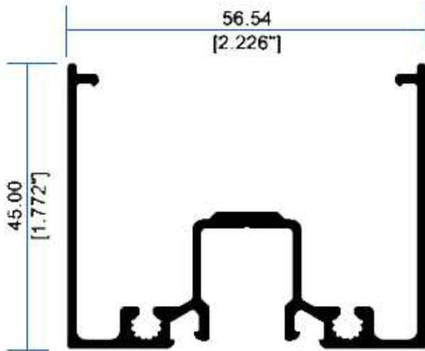
12504 Bolsa
