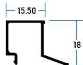
1432 Junquillo Extrecho
