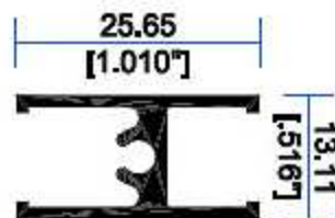
11203 Intermedio
