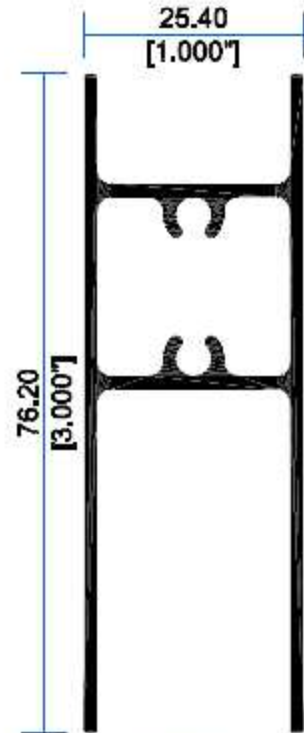
9959 Zoclo Pueta Duo
