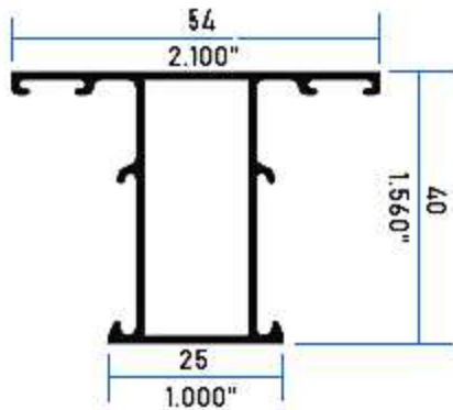
11400 Pilastra Lisa Ventana
