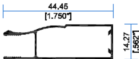
11046 Marco Semilujo 1 3/4"
