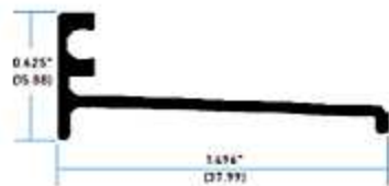
79742 Guia Nueva
