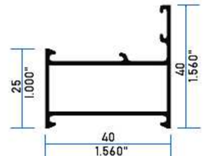
11402 Cercos Lisa Ventana
