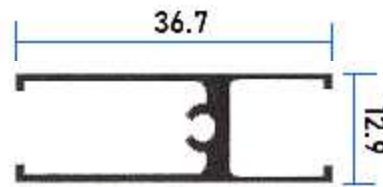
311044 Zoclo Cabezal
