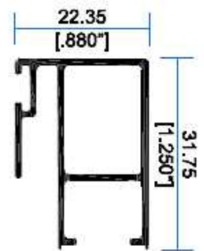
9954 Traslape Ventana
