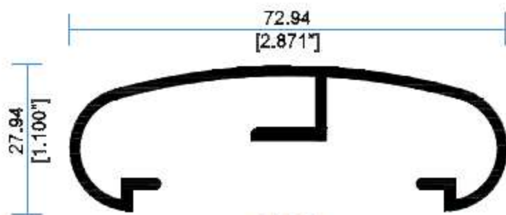
9366 Pasamano Ovalado
