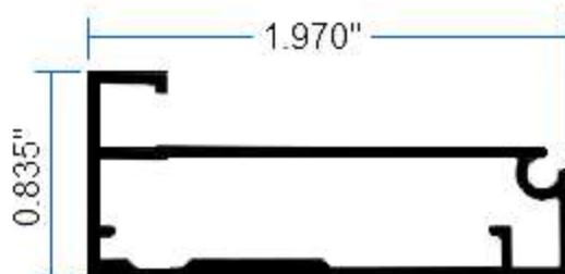
10701 Puerta Grande
