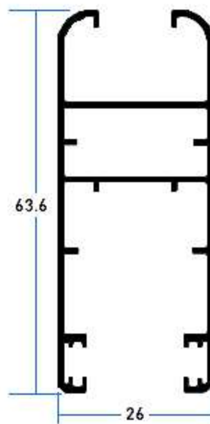
10512 Cerco
