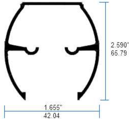
10468 Riel Superior 6mm Redondo
